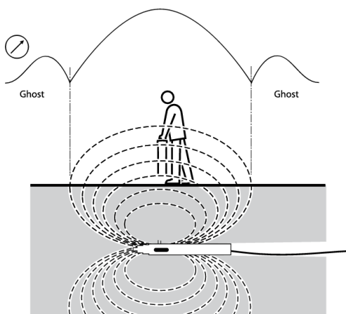
Obrázek 9.8 Vyhledání sondy
