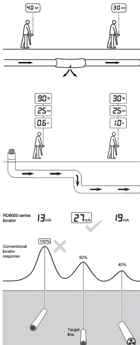
Obr. 6.4 - 6.6 Provádění měření proudu
