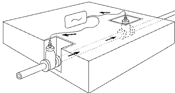
Obrázek 7.5: Vytváření oboustranných spojů
