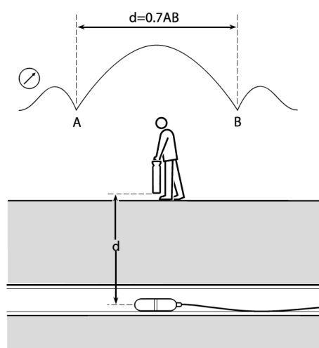
Obrázek 9.9: Výpočet hloubky sondy
