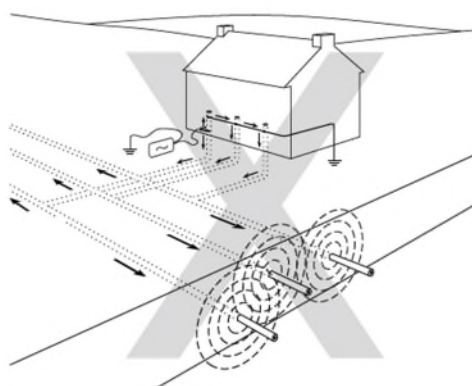
Obrázky 7.1 – 7.4: Nulování sítě a rušení signálu
