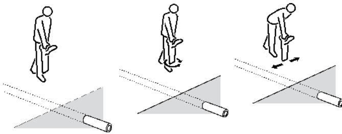
Obrázek 5.2: Přesné vyhledání cílového vedení
