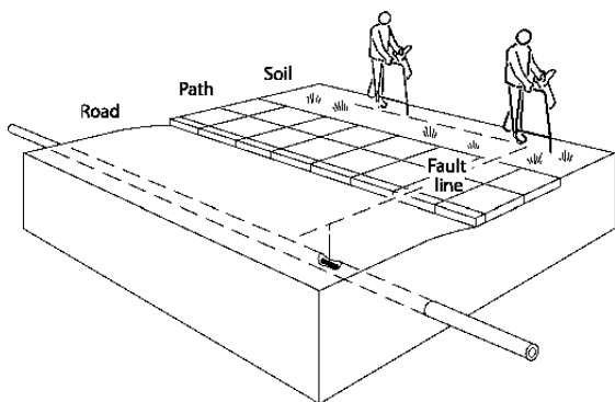
Obrázek 8.2: Lokalizace poruch pomocí lokátoru a A-rámu
