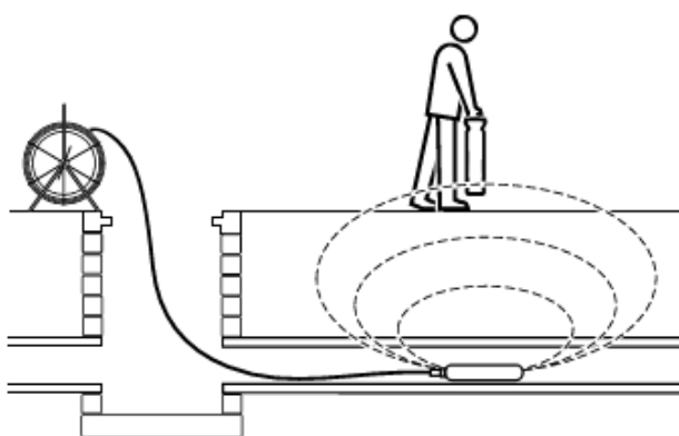
Obrázek 9.7 Nasazení sondy
